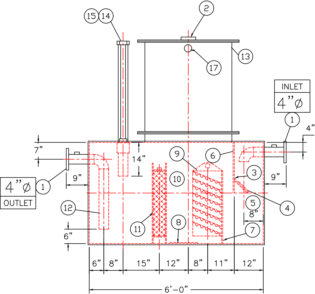
ELEVATION
