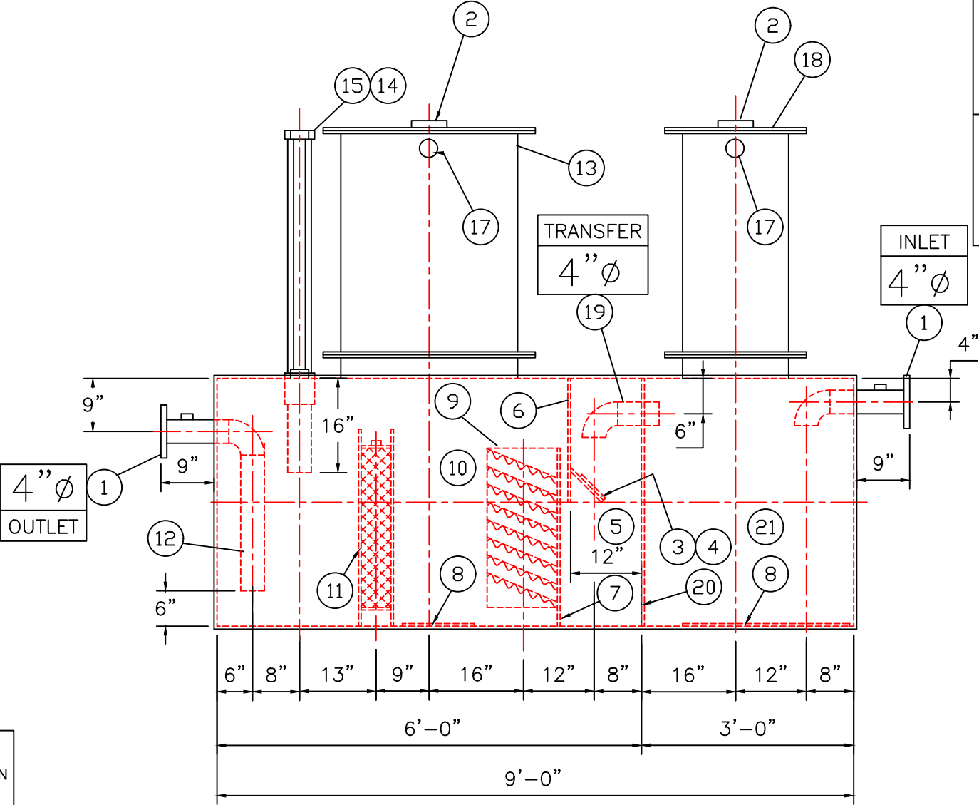
ELEVATION
