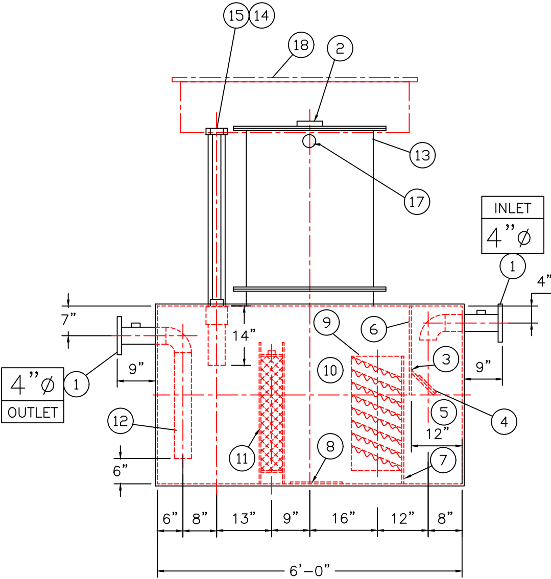
ELEVATION
