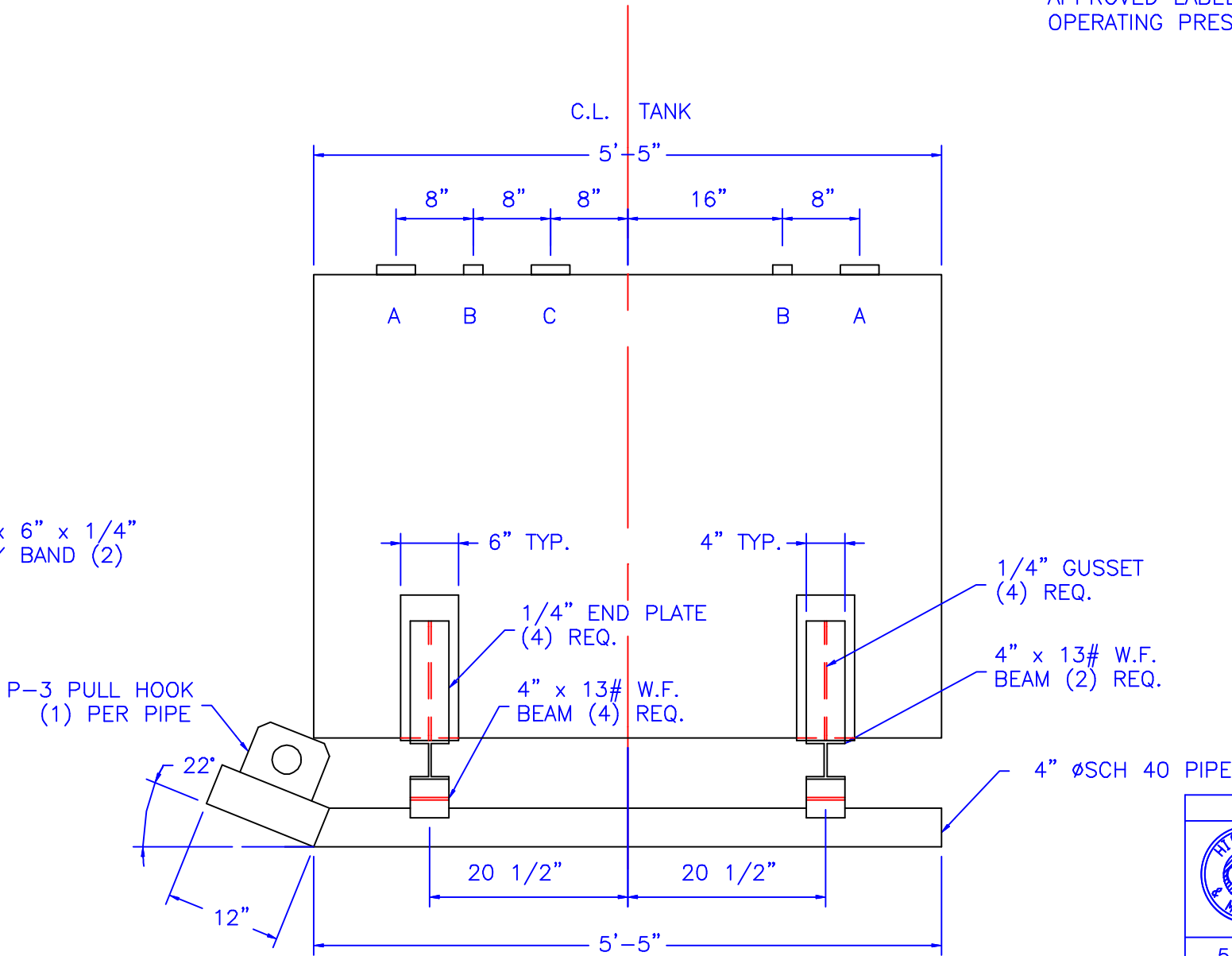
ELEVATION
