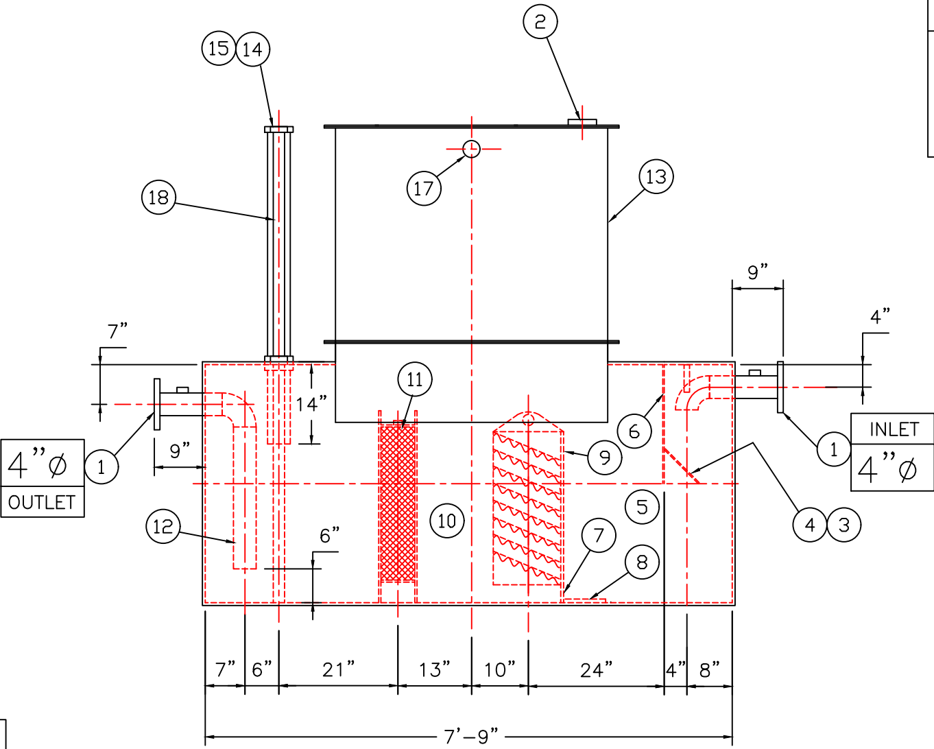
ELEVATION
