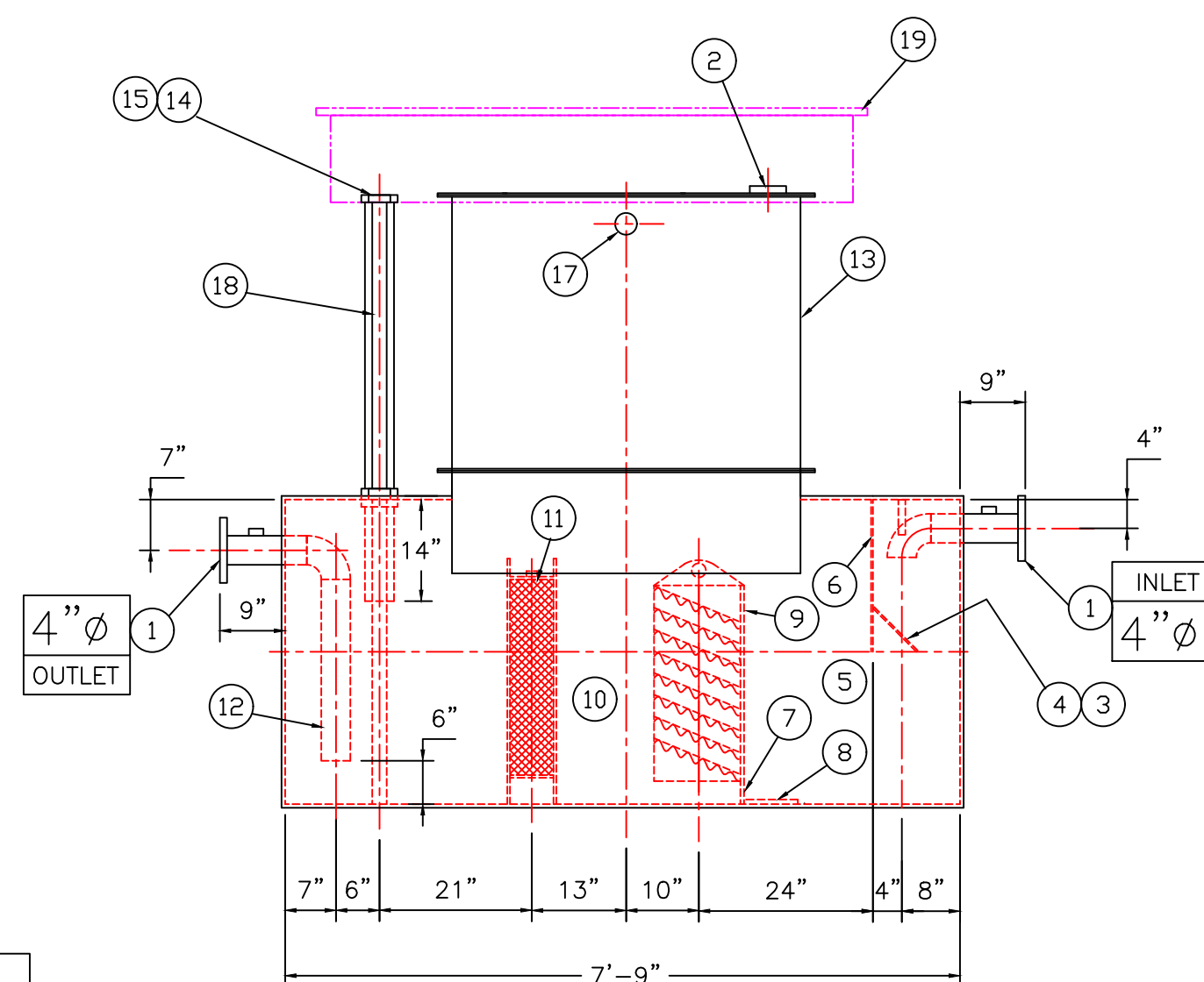
ELEVATION
