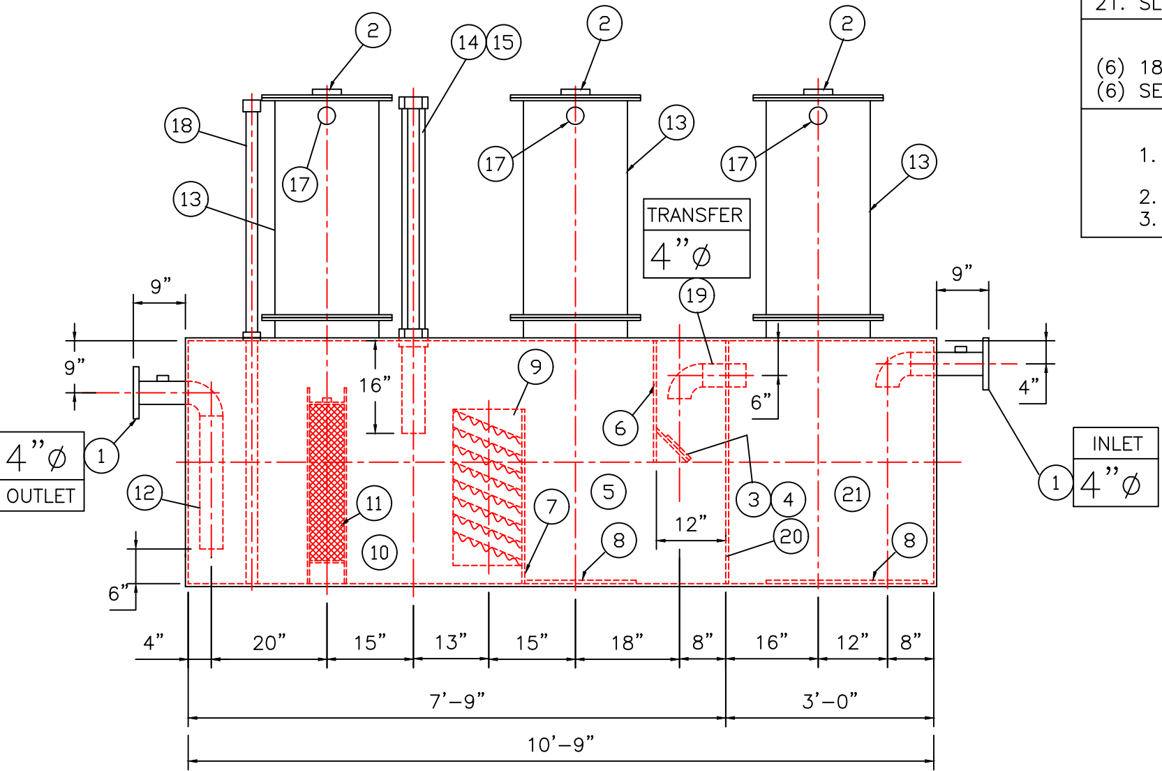
ELEVATION
