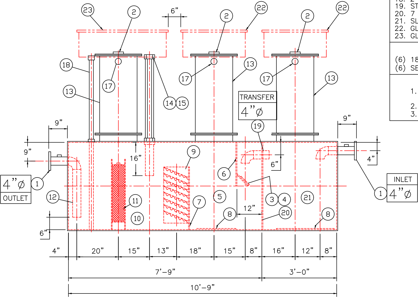
ELEVATION
