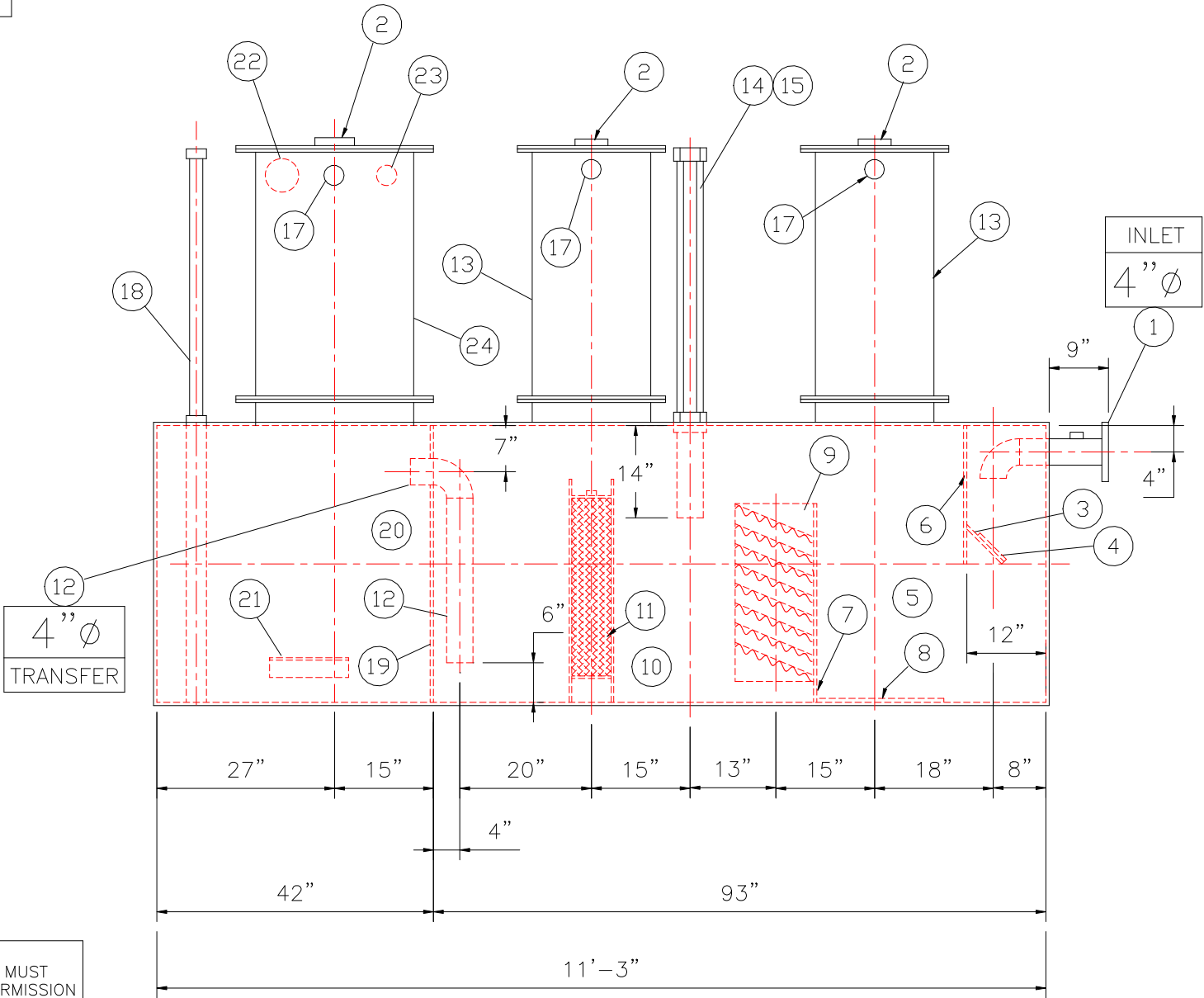
ELEVATION
