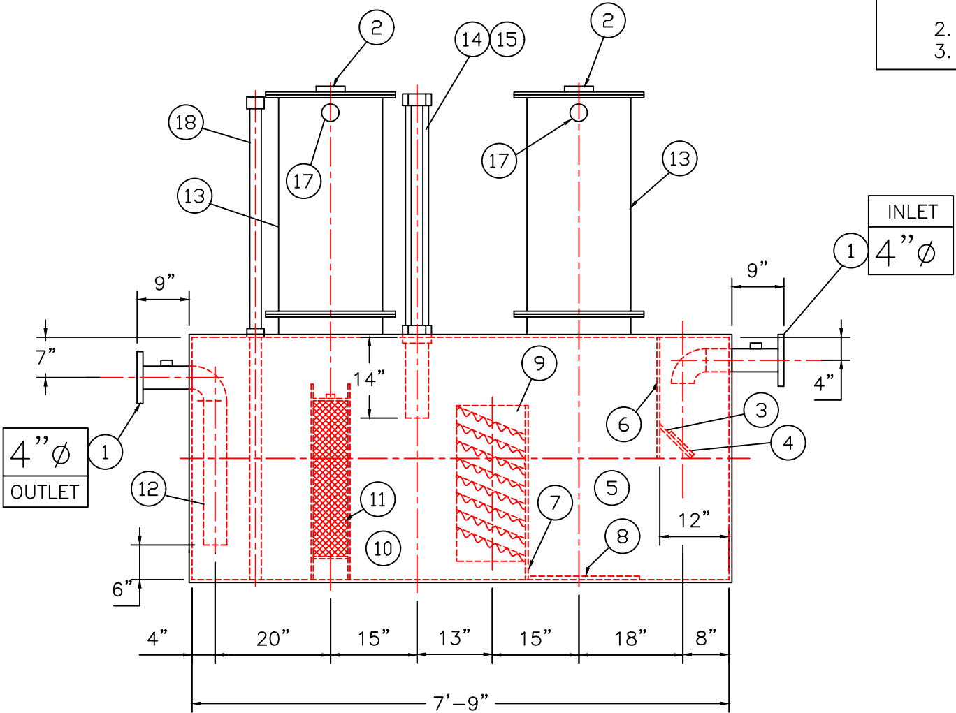
ELEVATION
