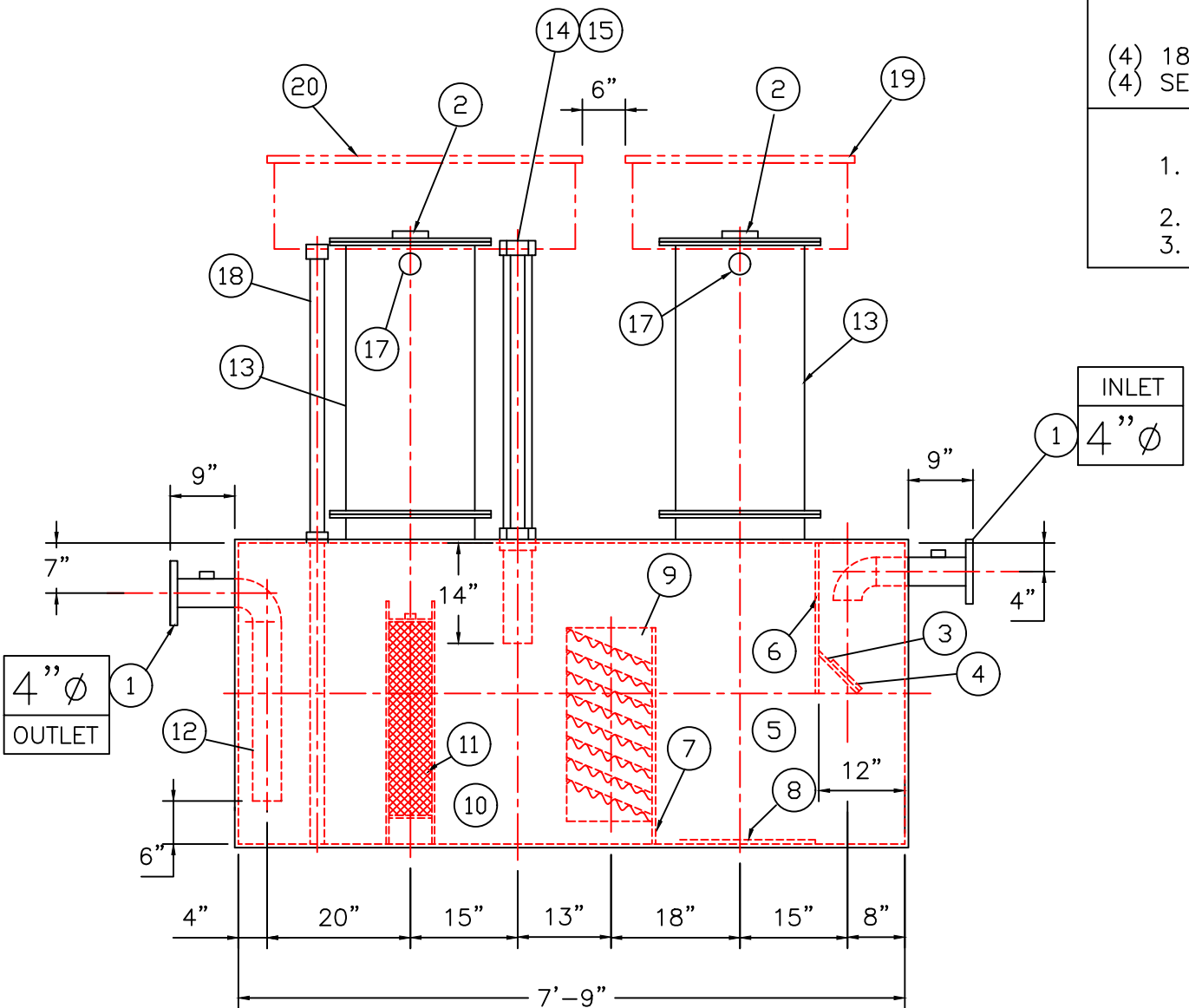
ELEVATION
