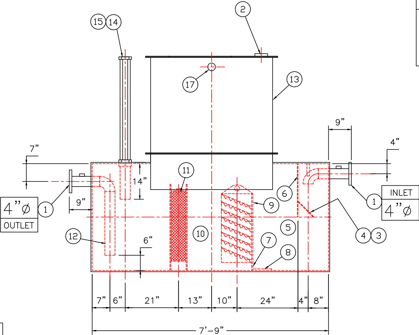
ELEVATION
