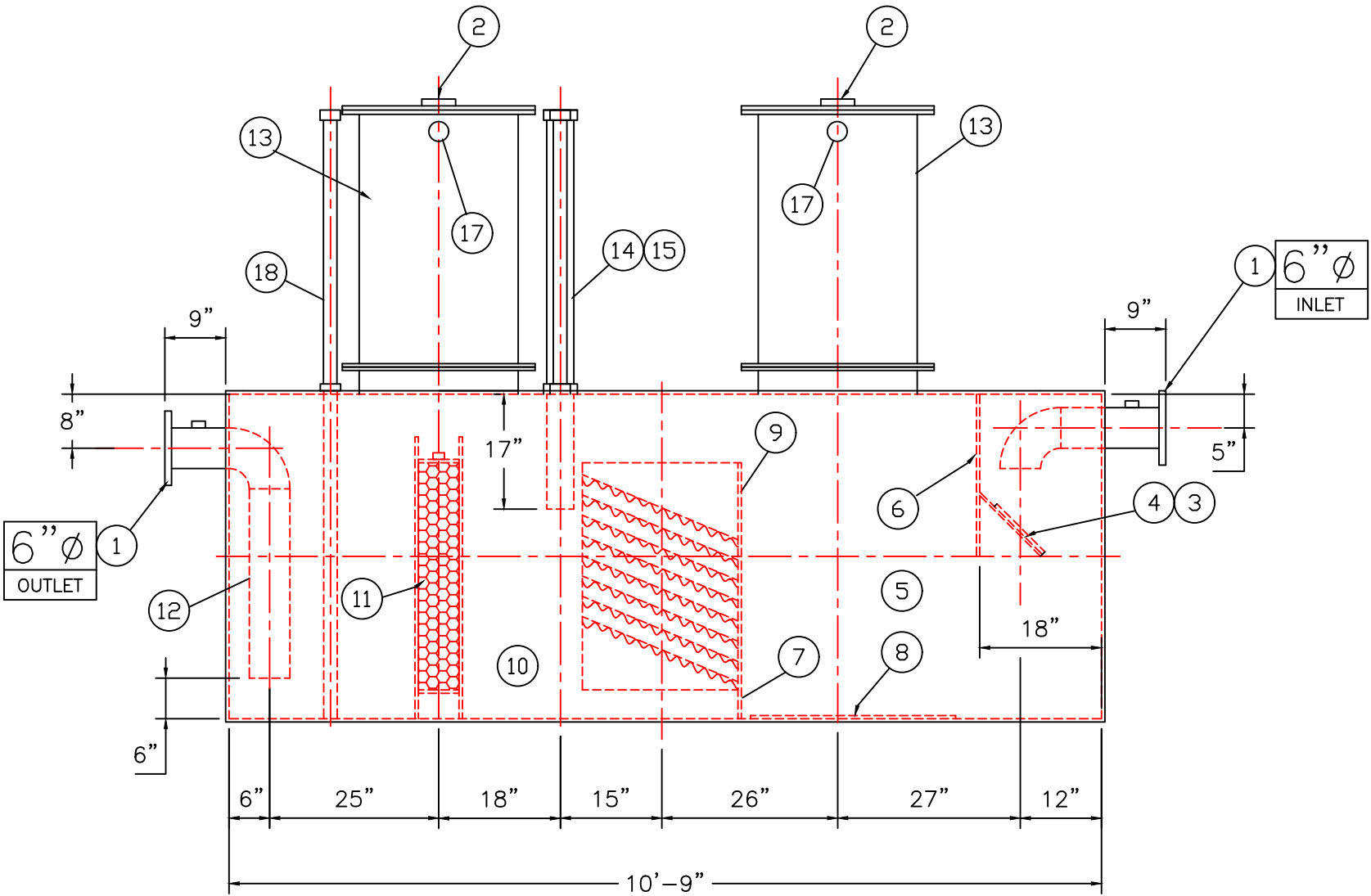
ELEVATION
