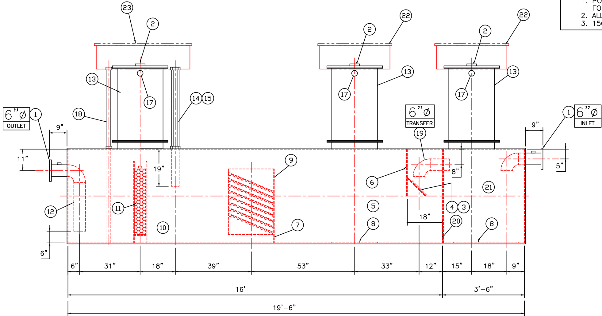
ELEVATION
