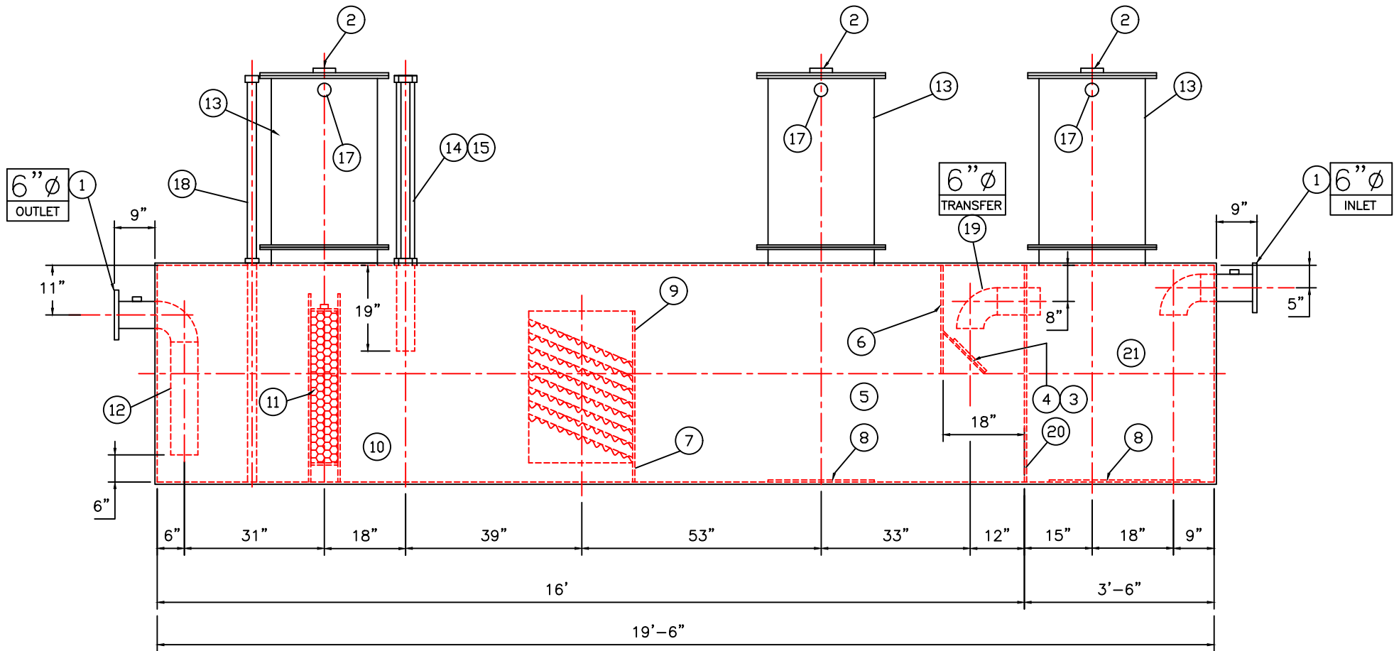
ELEVATION
