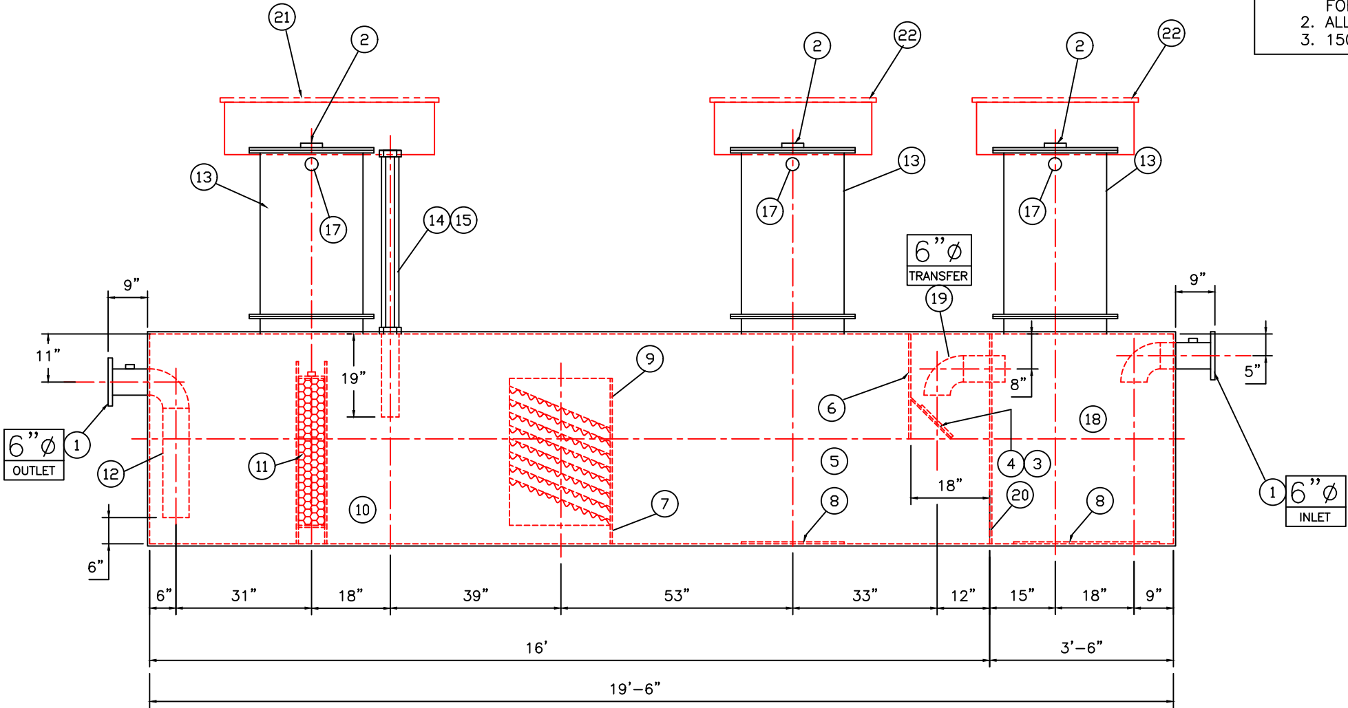
ELEVATION
