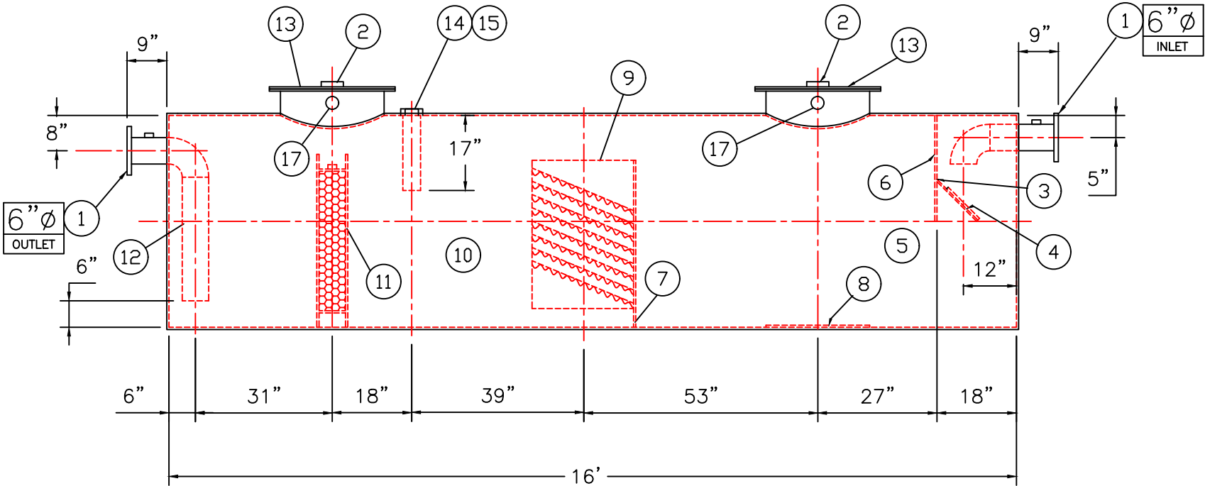
ELEVATION
