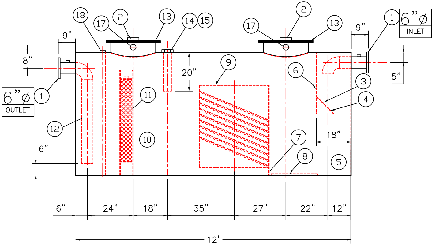
ELEVATION
