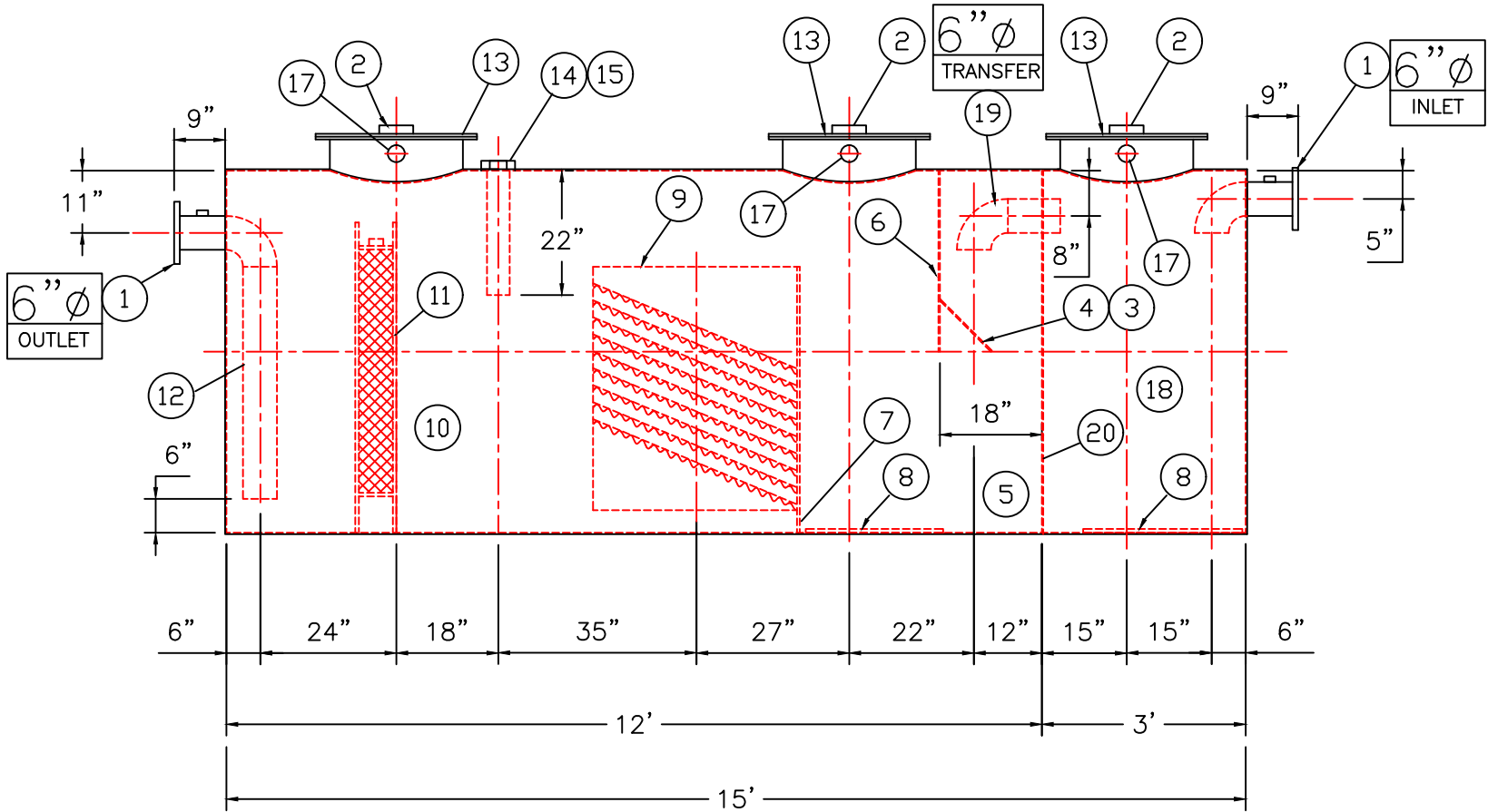
ELEVATION
