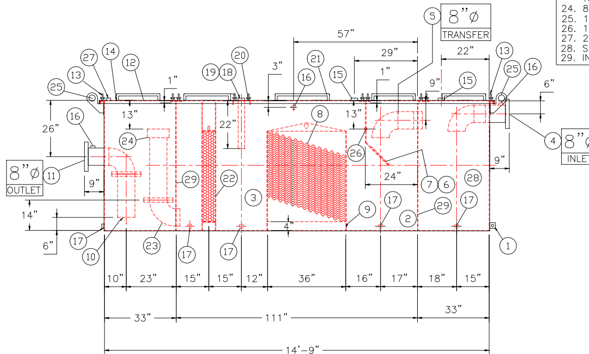
ELEVATION
