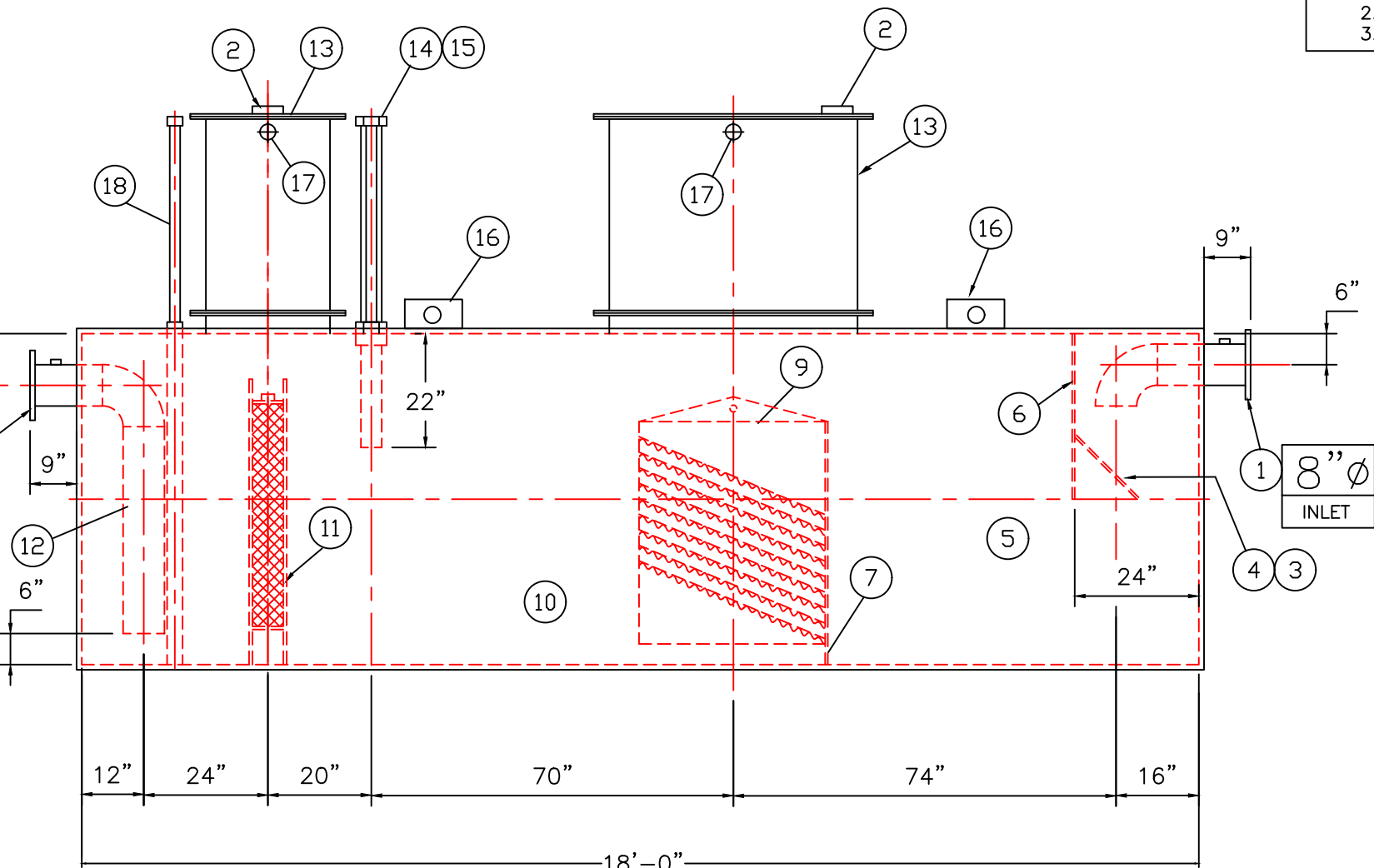
ELEVATION
