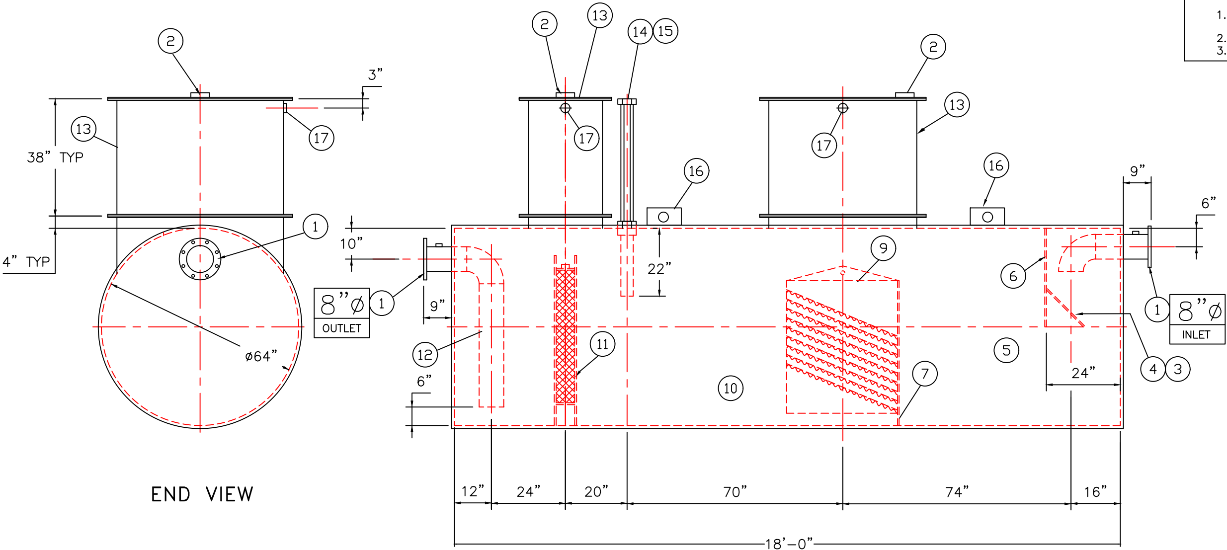
ELEVATION
