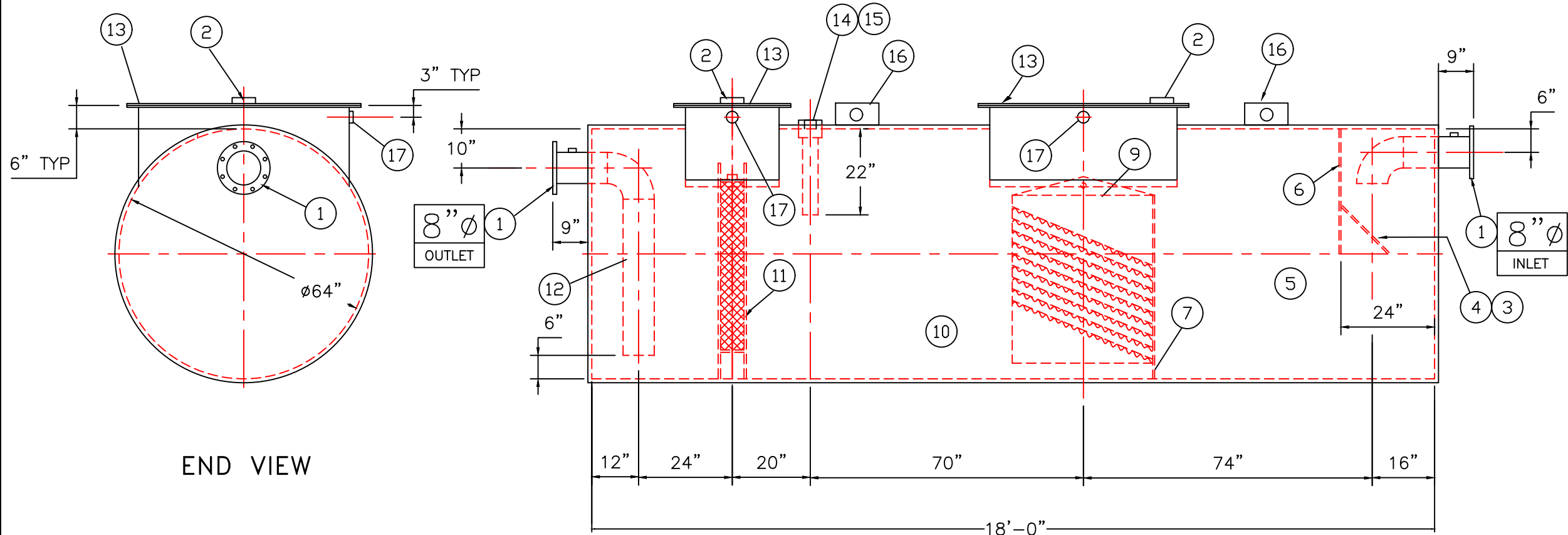
ELEVATION
