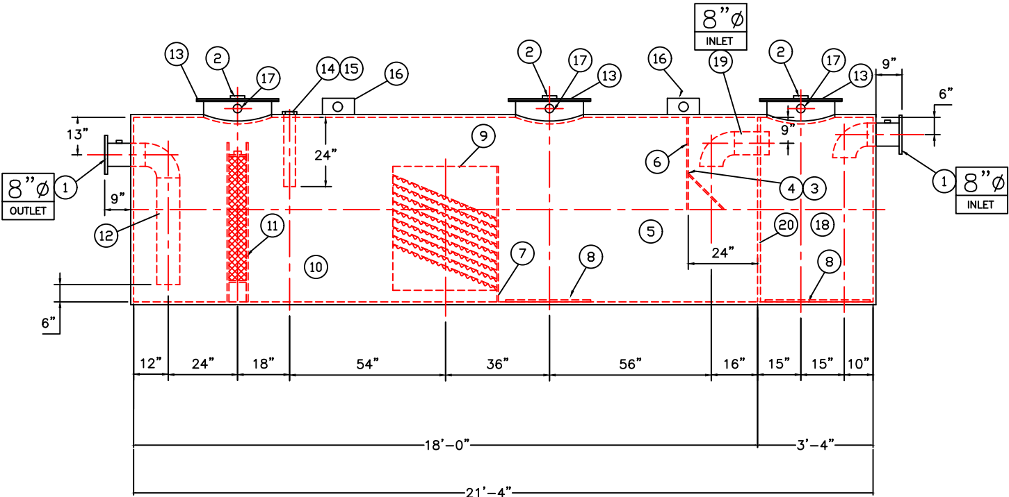
ELEVATION
