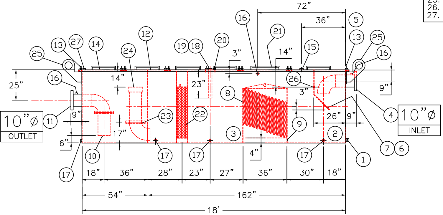
ELEVATION
