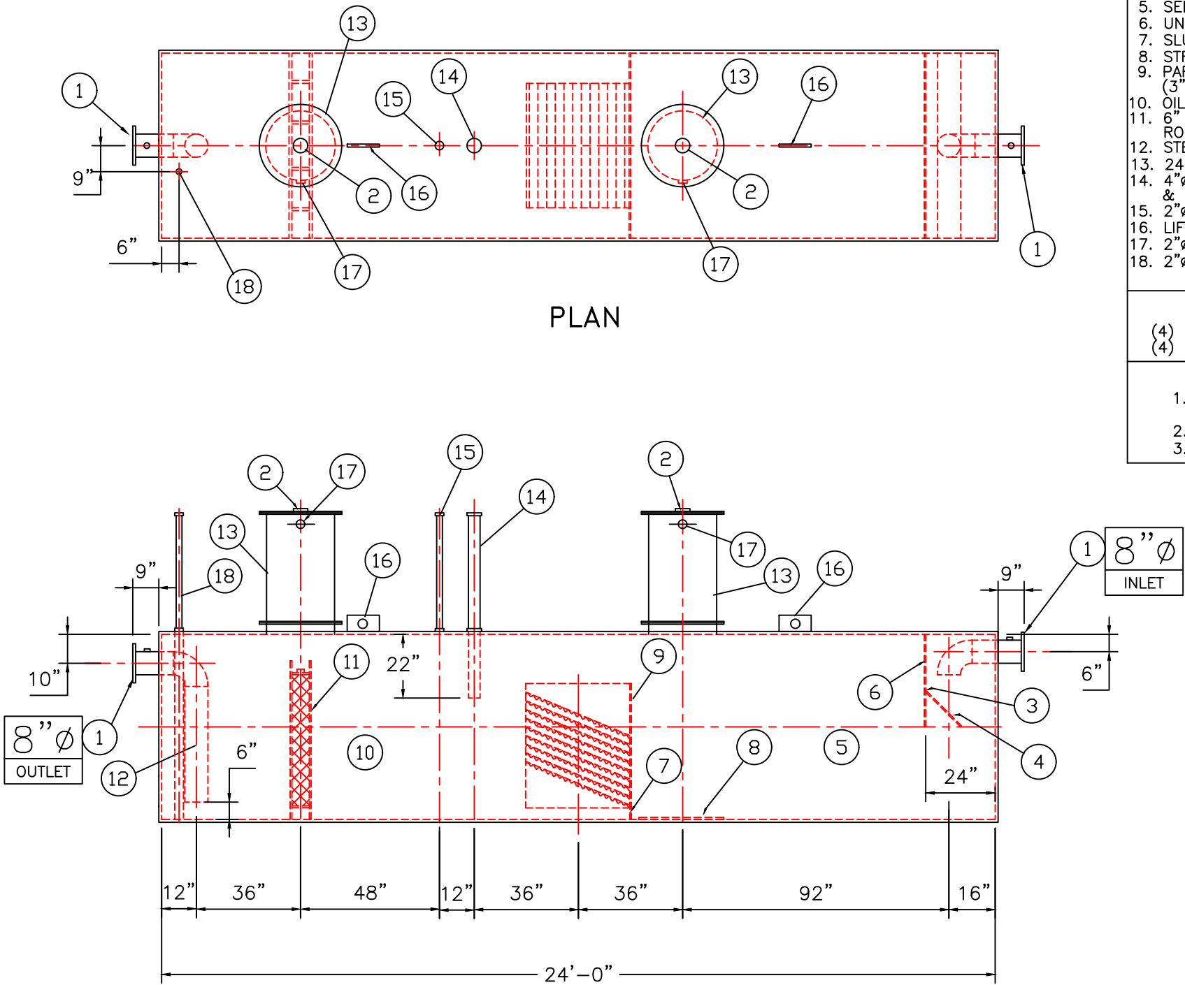
ELEVATION
