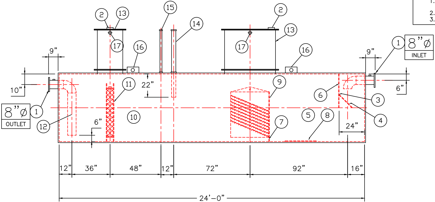
ELEVATION
