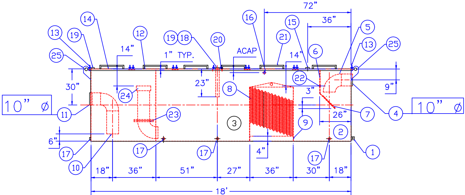
ELEVATION
