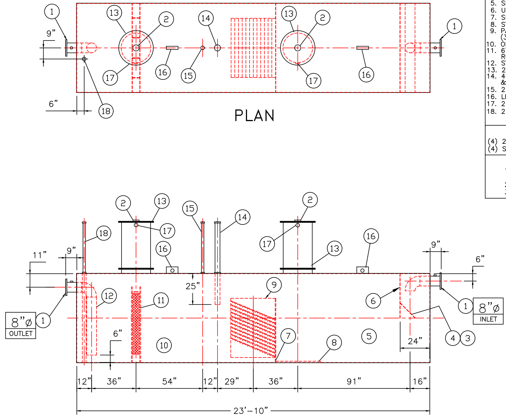
ELEVATION
