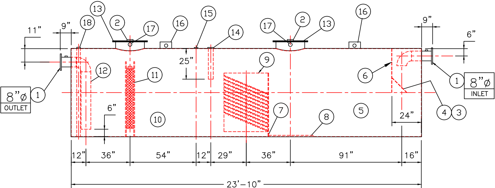
ELEVATION
