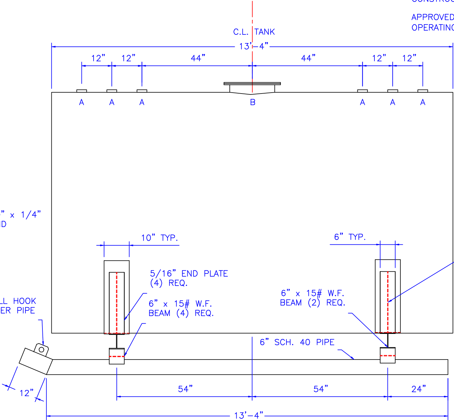
ELEVATION
