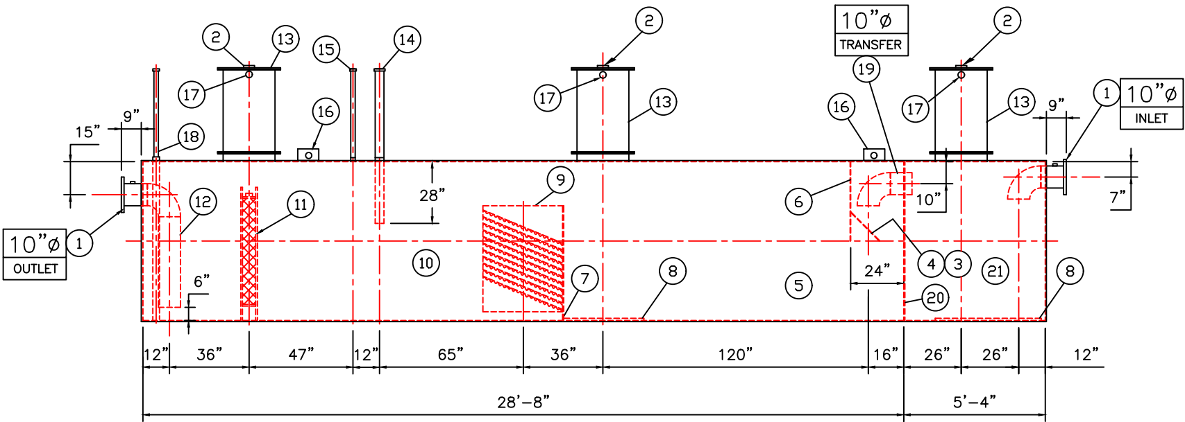
ELEVATION
