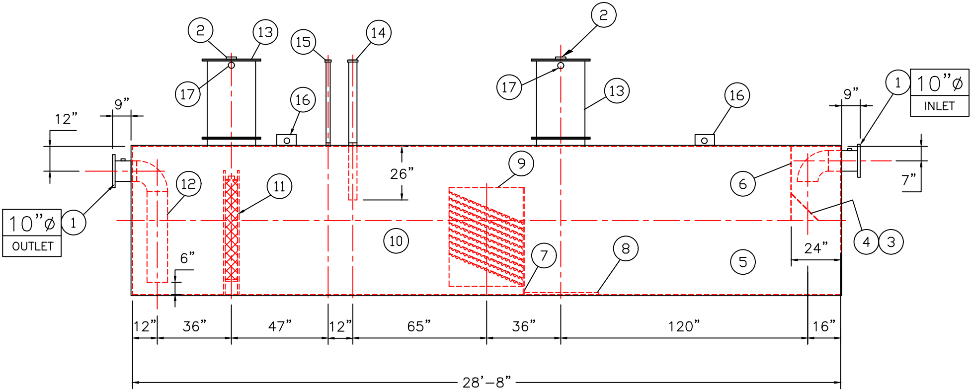
ELEVATION
