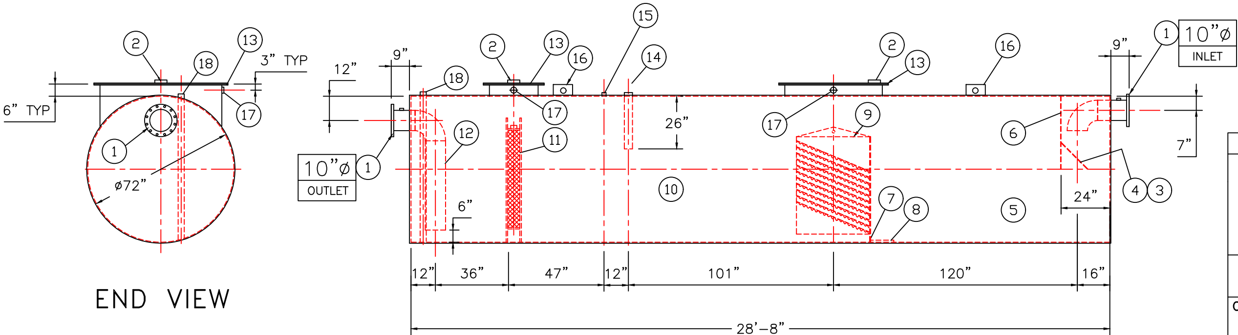
ELEVATION
