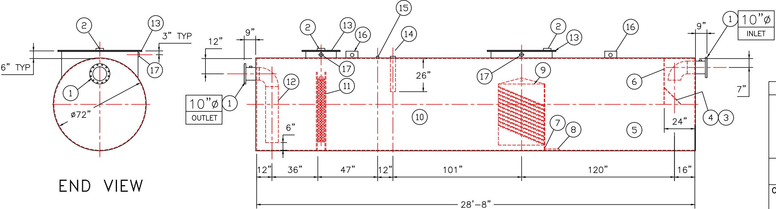
ELEVATION
