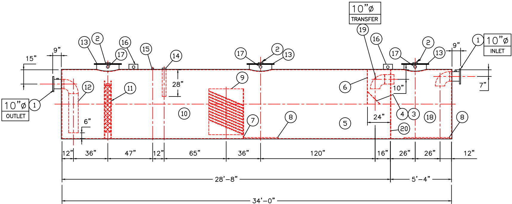
ELEVATION
