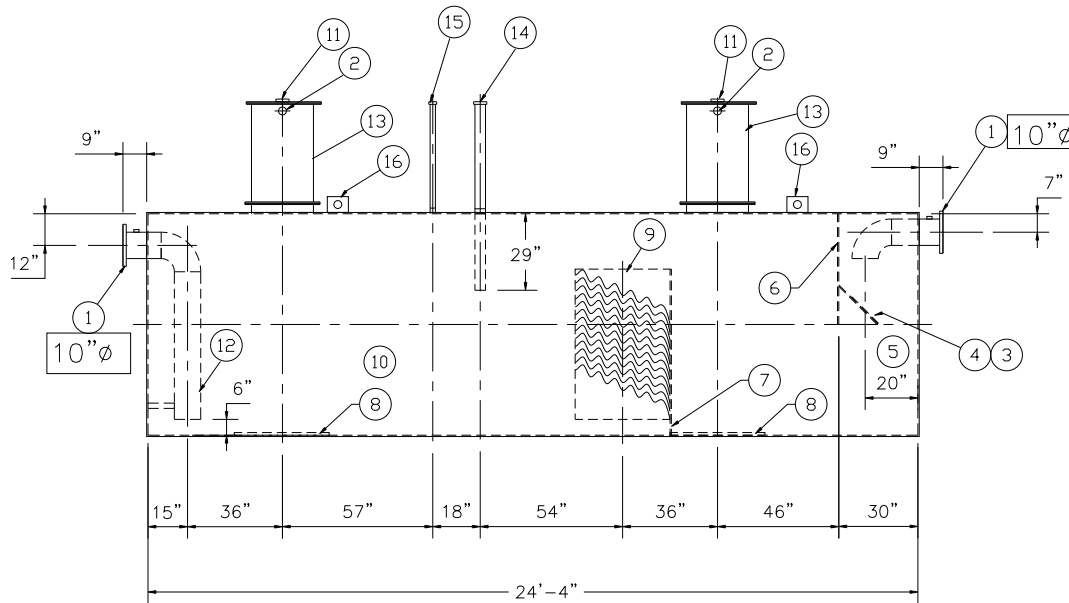
ELEVATION
