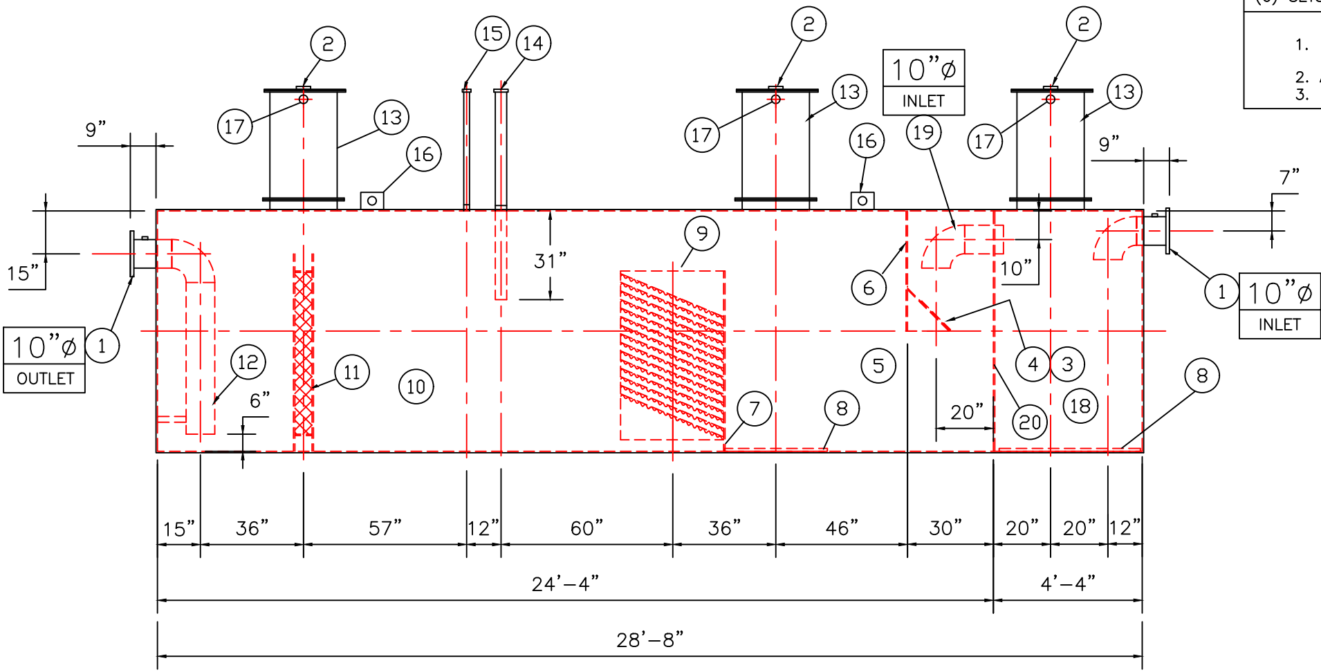
ELEVATION
