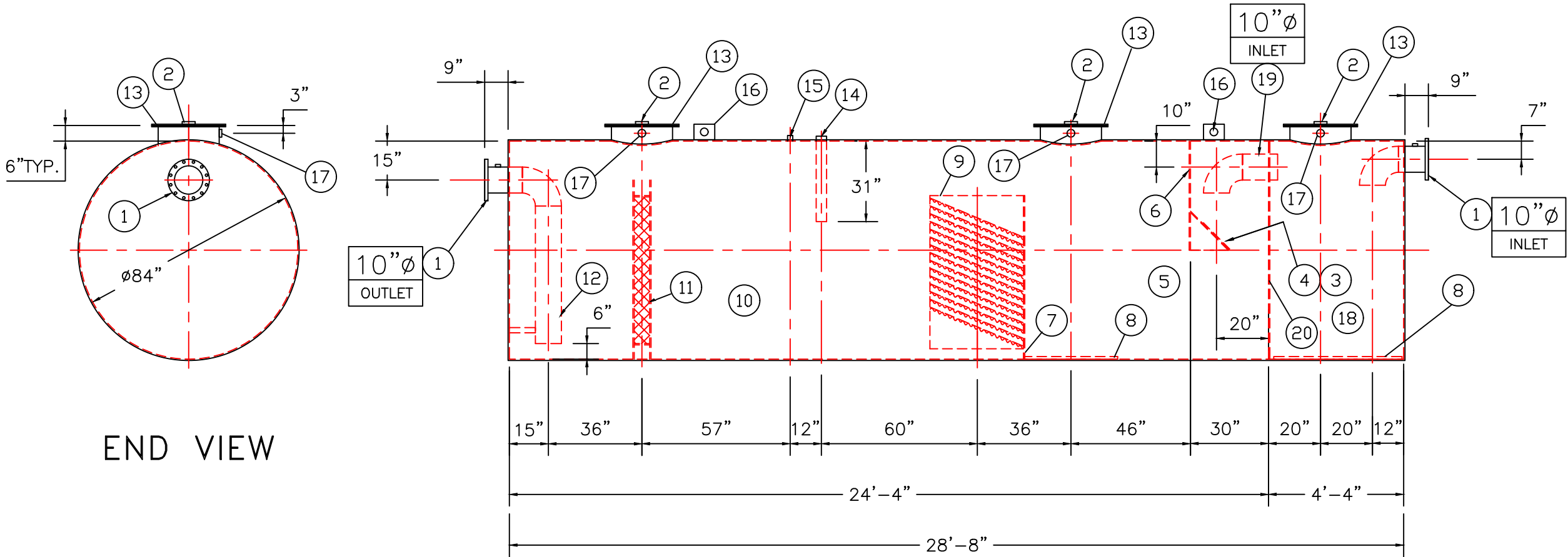
ELEVATION
