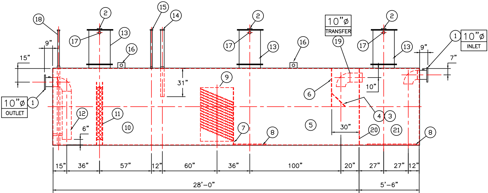
ELEVATION
