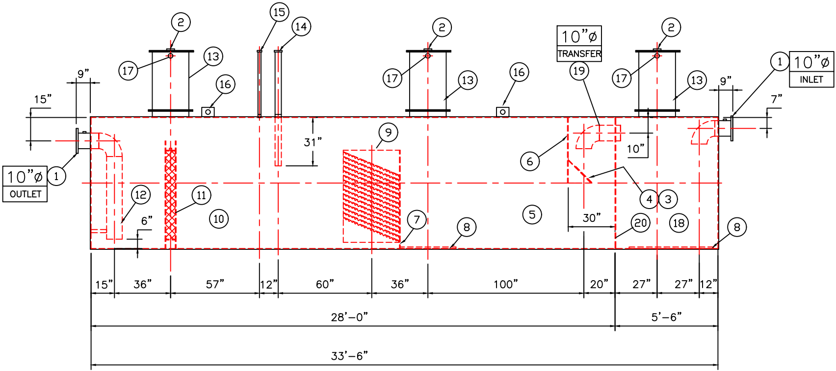
ELEVATION
