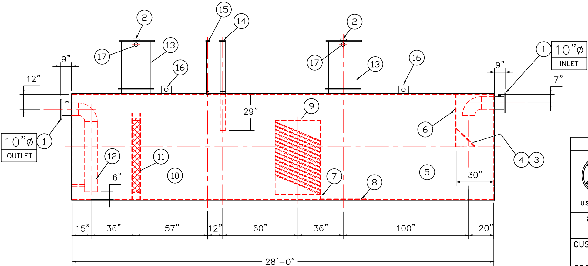
ELEVATION
