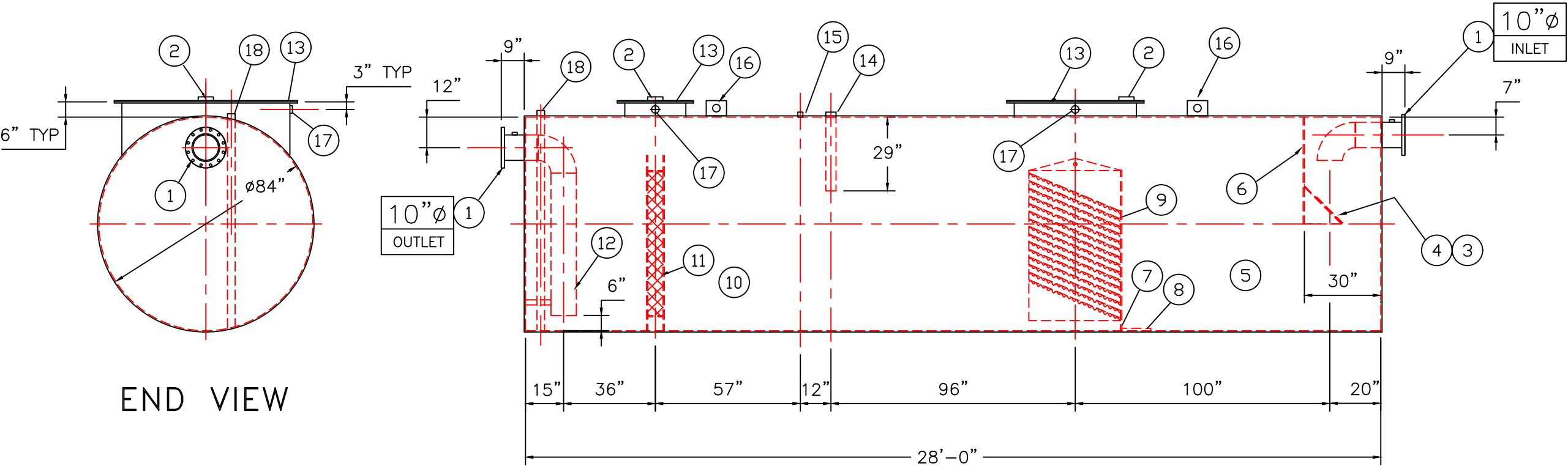
ELEVATION
