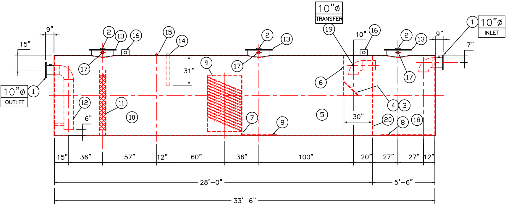
ELEVATION
