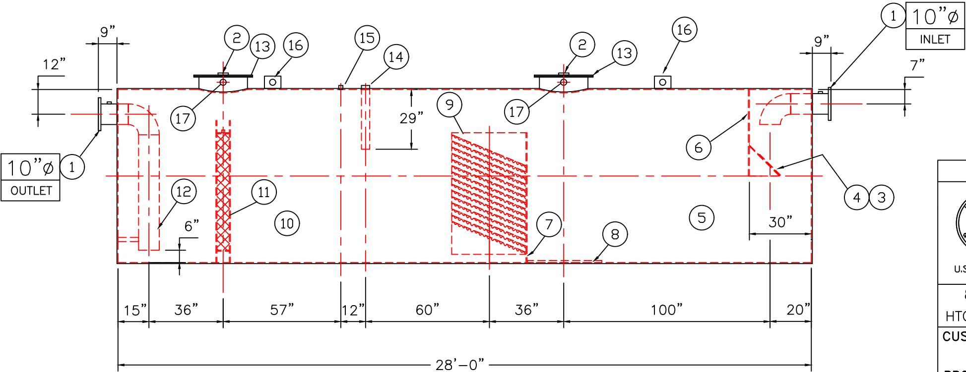
ELEVATION
