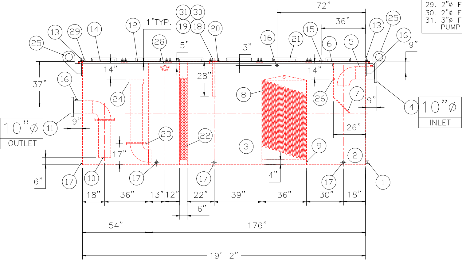
ELEVATION
