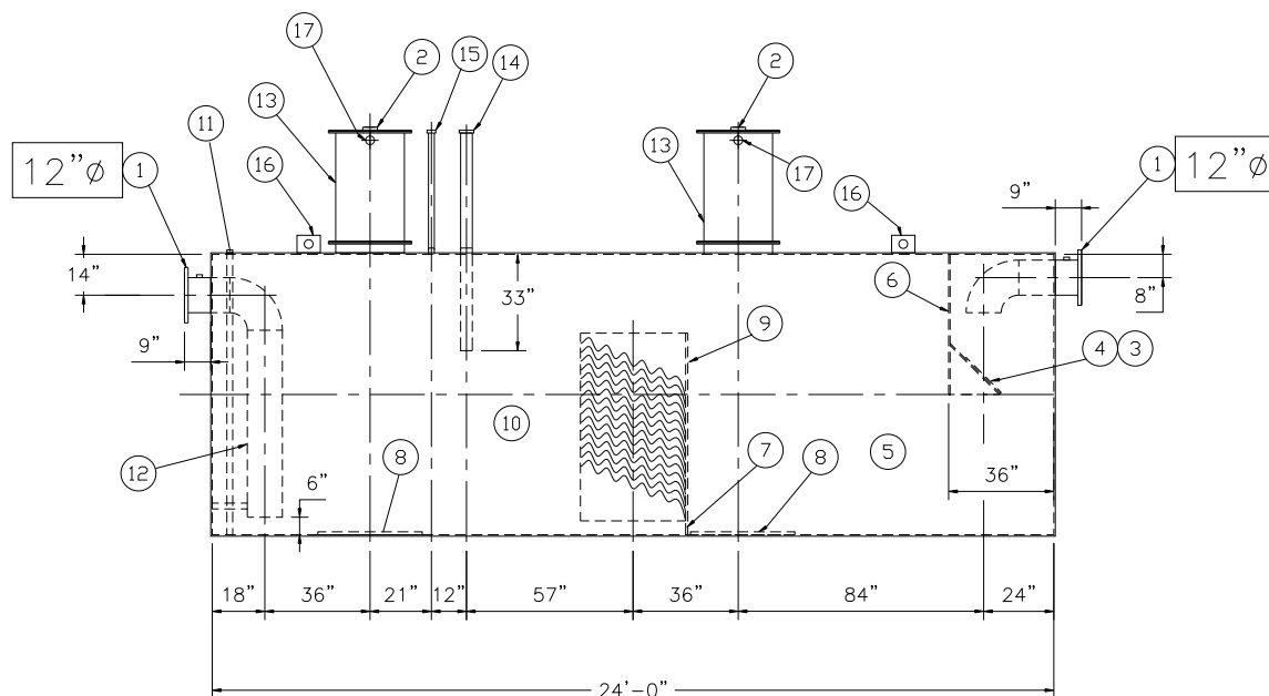
ELEVATION
