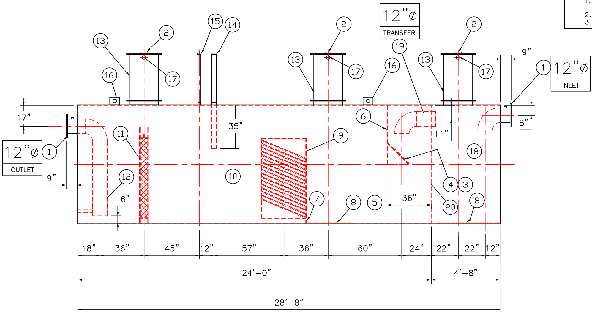
ELEVATION
