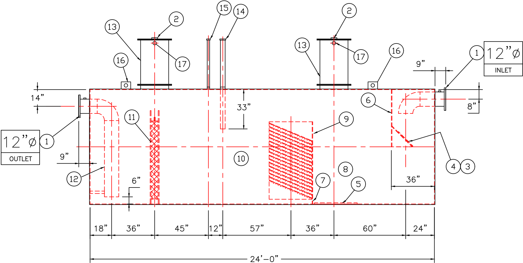
ELEVATION
