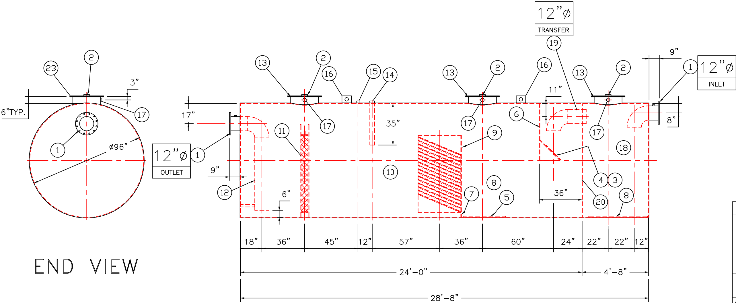
ELEVATION
