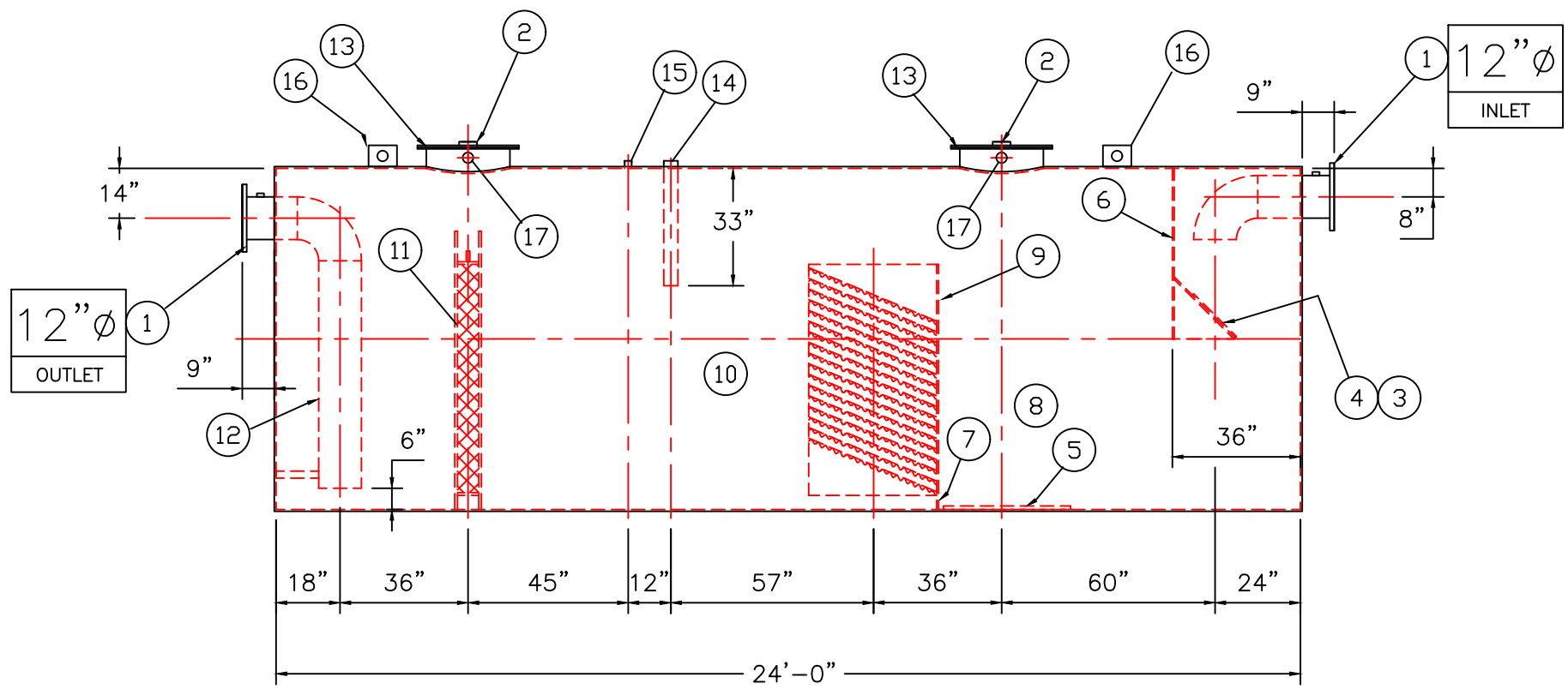
ELEVATION
