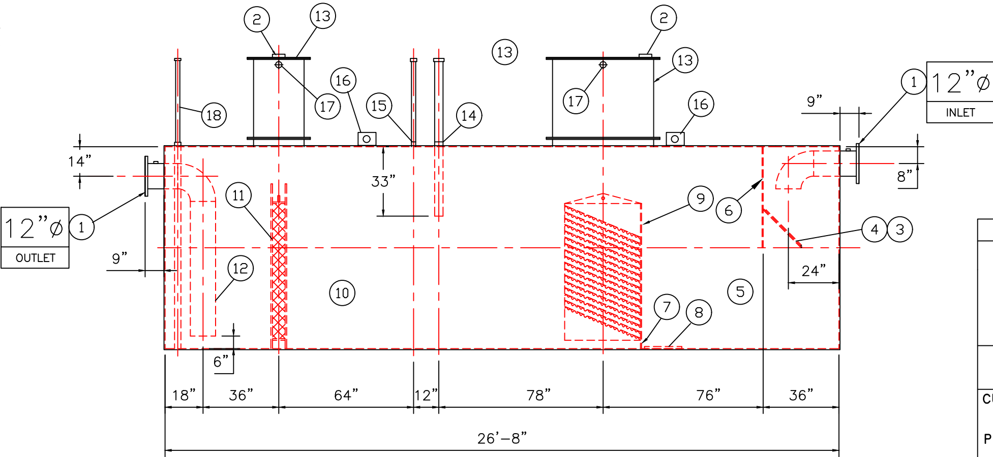
ELEVATION
