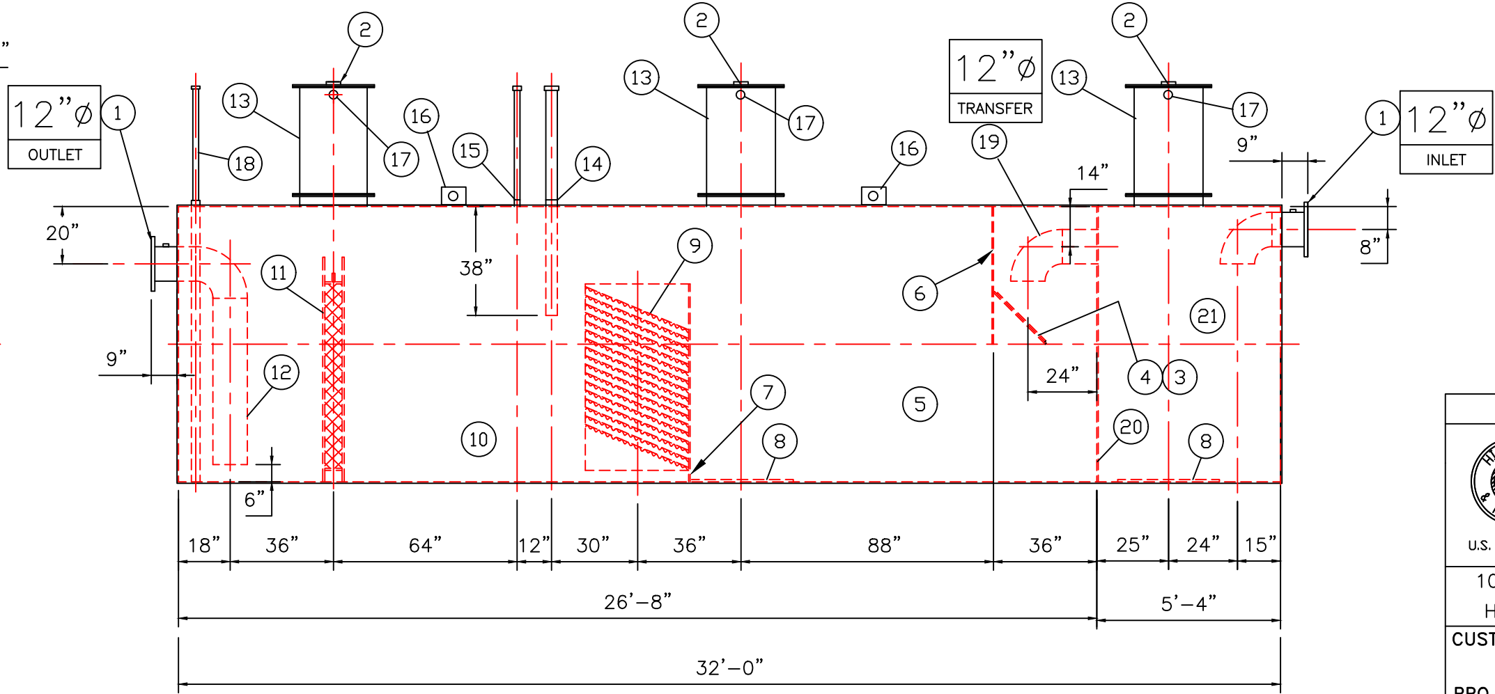
ELEVATION
