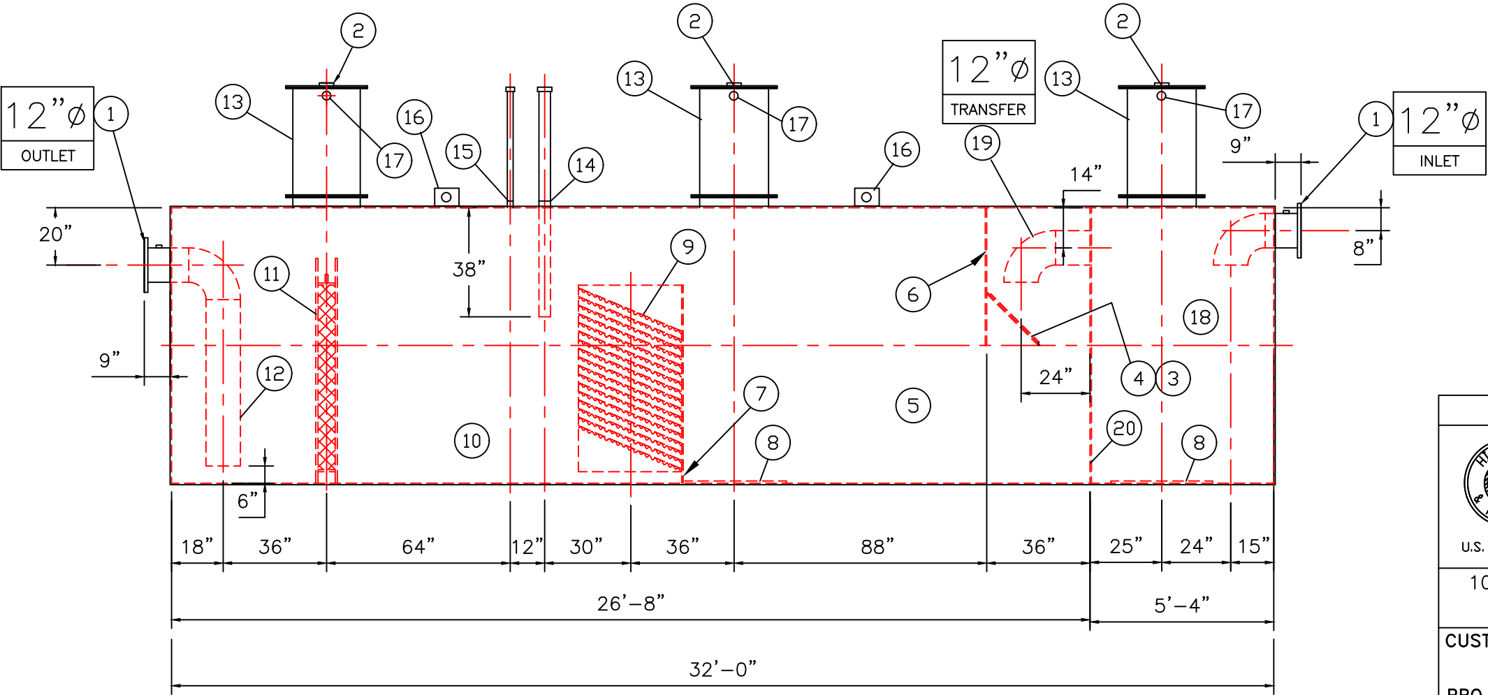
ELEVATION
